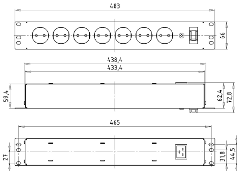
Рисунок 2. Монтажно-габаритные размеры блока розеток REC- S716A
