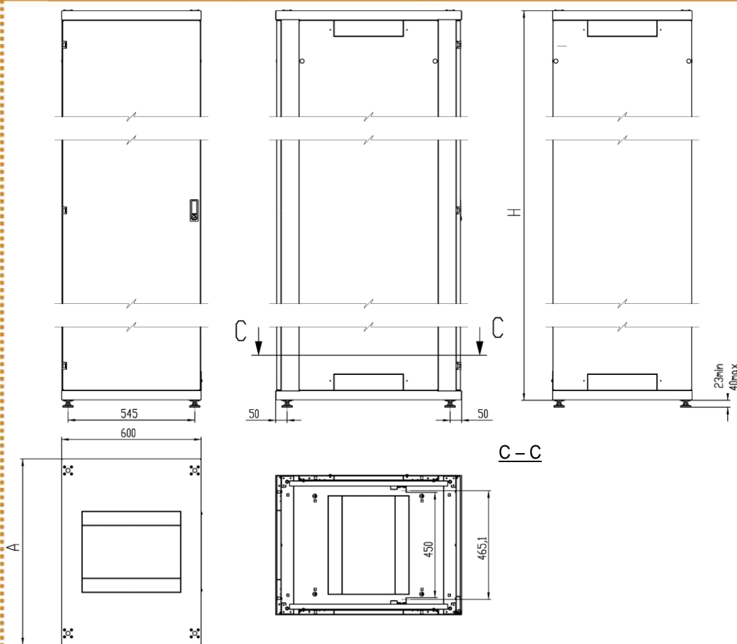
Рисунок 3: Монтажно-габаритные чертежи
